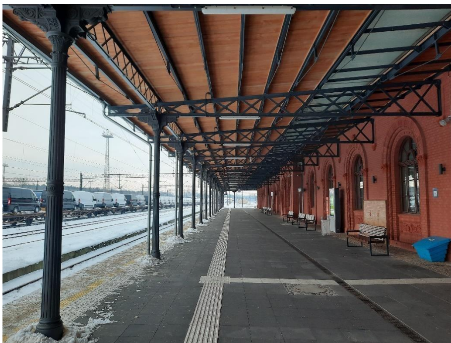
Ryc. 15. Wiatą peronowa na dworcu w Węglińcu. Fot. P. Zubrzycki.
