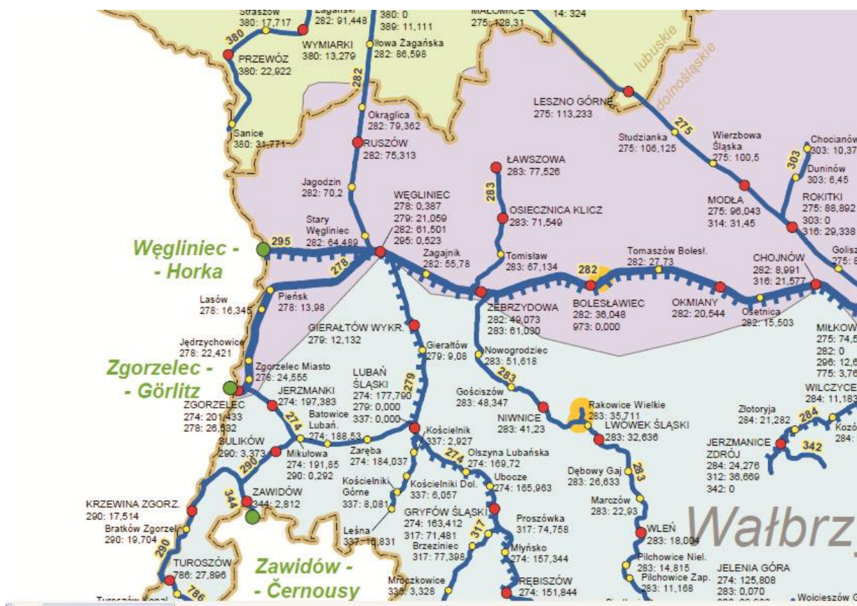
Rys. 16 Schemat przebiegu linii kolejowych na terenie Gminy Węgliniec
